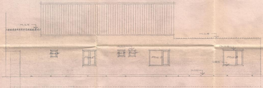
Facade mod nord 1:50
