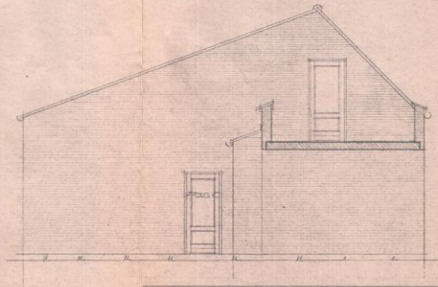
Gavl mod syd 1:50
