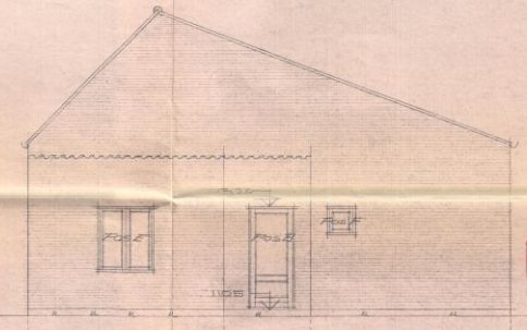
Gavl mod vest 1:50
