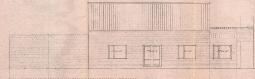
Facade mod øst 1:50
