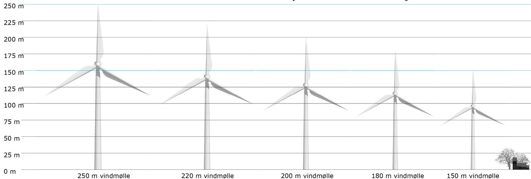
Figur 6-4. Eksempler på trevingede vindmøller.
