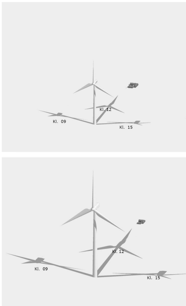
Figur 7-2. Illustration af skyggekast fra vindmølle, henholdsvis maksimal totalhøjde 150 og 250 m. Forårs- og efterårsjævndøgn Kl. 09 | 12 | 15. Højere vindmøller medfører større skyggekast i nærområdet.
