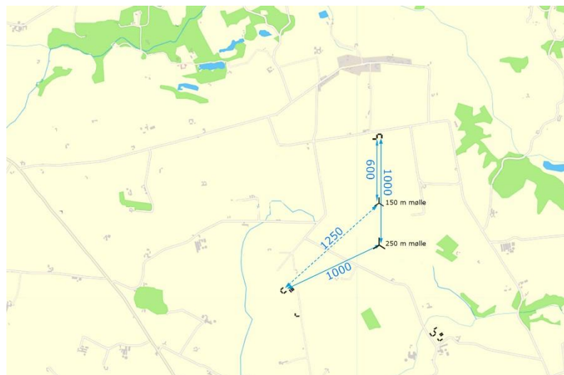
Figur 6-19. Illustration af et teoretisk eksempel, hvor en 150 meter høj vindmølle er placeret 600 m fra nærmeste nabobeboelse og 1.250 m fra en anden beboelse. Hvis den 150 meter høje vindmølle skal udskiftes med en vindmølle på 250 meters højde, skal møllen flyttes 1.000 meter væk fra nærmeste nabobeboelse. Vindmøllen er i eksemplet flyttet mod syd, og kommer derfor til at ligge tættere på den anden beboelse end den 150 meter høje vindmølle gjorde. Den visuelle påvirkning vil derfor være større, selvom minimumsafstanden er overholdt.
